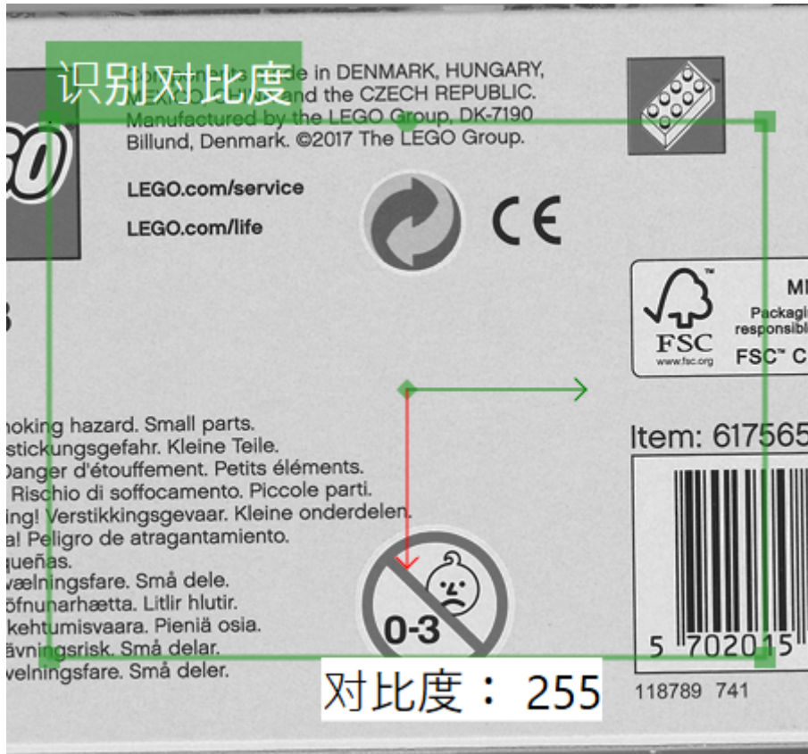
图 152: 识别对比度工具的图像 GUI。
