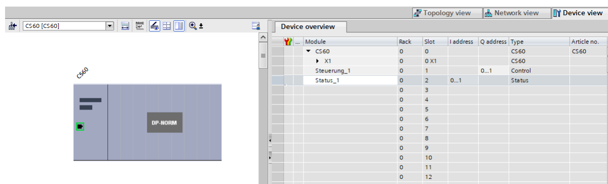
图 216: 将模块添加到 CS-60/ID-600 插槽
