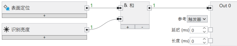
图 168: 不同工具的逻辑组合。
