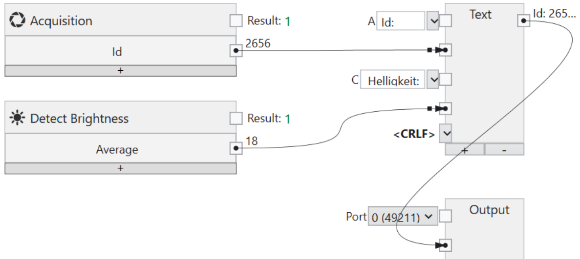
图 200: 用于 TCP/IP 输出电流的文本组合。
