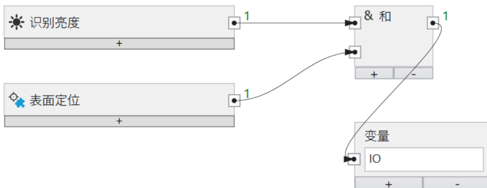
图 187: 不同工具的逻辑组合。
