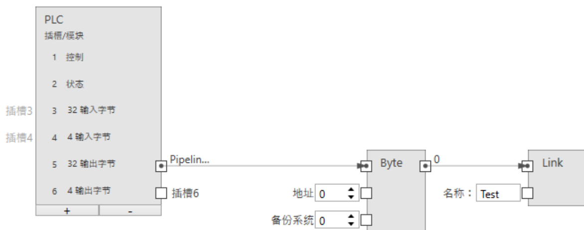
图 54: 字节输入。
