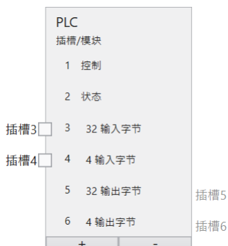
图 197: 具有六个模块的 PLC 节点。
