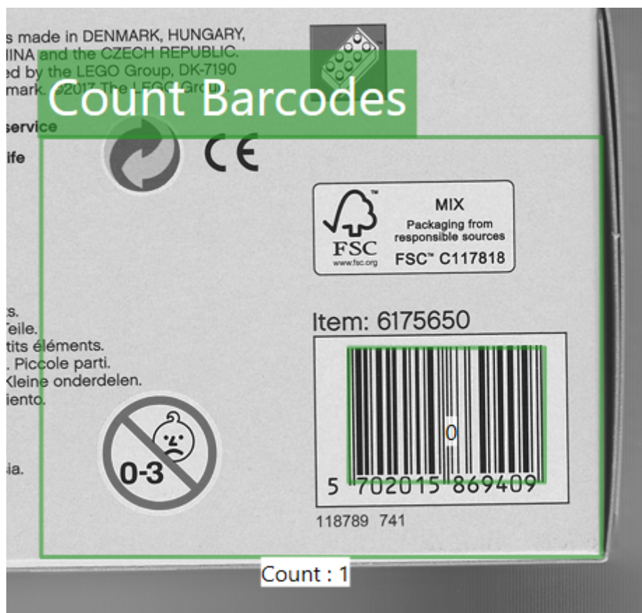
图 84: 条形码计数工具的图像 GUI。
