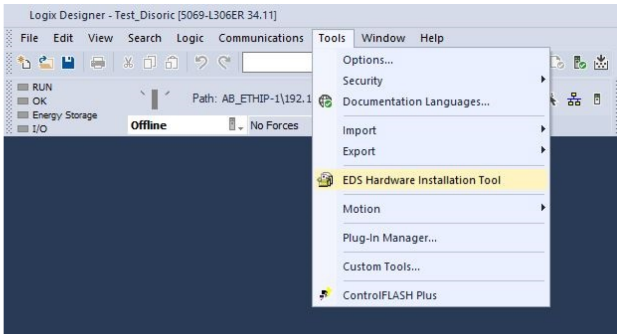
图 217: 找到 CS-60/ID-600 的 EDS 文件
