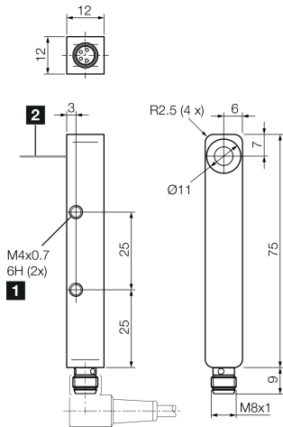
1) Alésage / Filetage (traversant) 2) Sortie sonore transducteur à ultrasons BK: noir BN: marron BU: bleu WH: blanc
