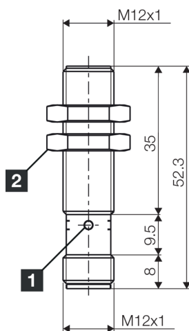
1) LED 4 x 90° (jaune) 2) Ouverture de clé 17 mm BK: noir BN: marron BU: bleu
