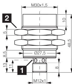
1) LED 4 x 90° (jaune) 2) Ouverture de clé 36 mm BN: marron BU: bleu WH: blanc
