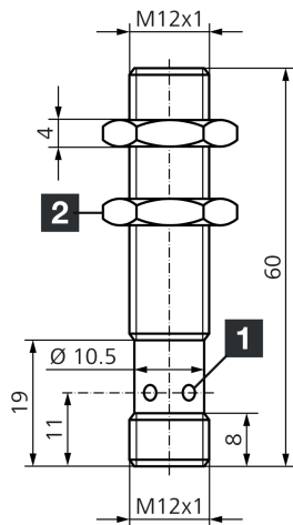
1) LED 4 x 90° (gelb) 2) Schlüsselweite 17 mm BK: schwarz BN: braun BU: blau
