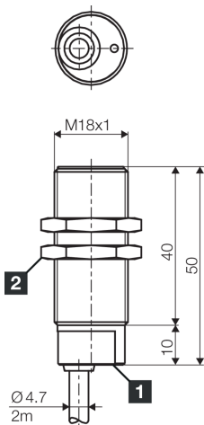
2) Schlüsselweite 24 mm
