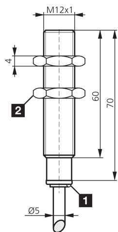
2) Schlüsselweite 17 mm
