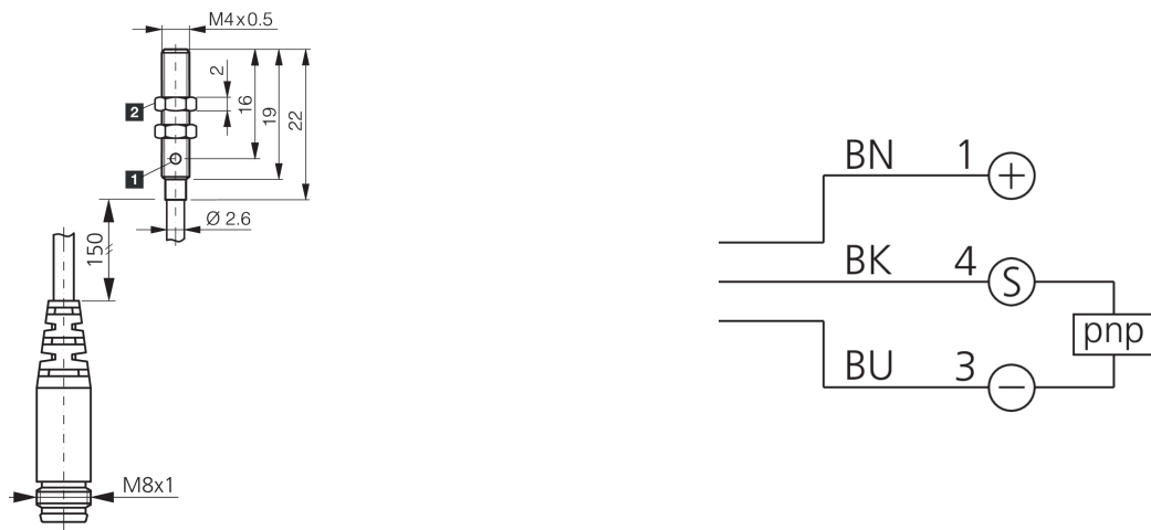
1) LED 2) Schlüsselweite 6 mm BK: schwarz BN: braun BU: blau
