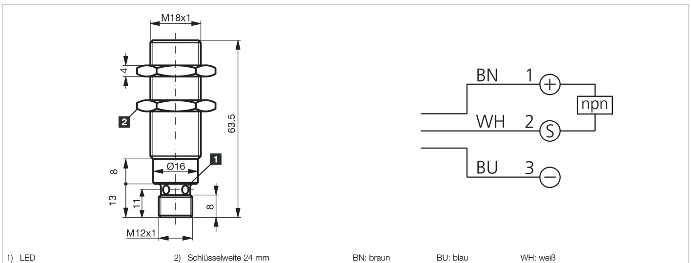
1) LED 2) Schlüsselweite 24 mm BN: braun BU: blau WH: weiß
