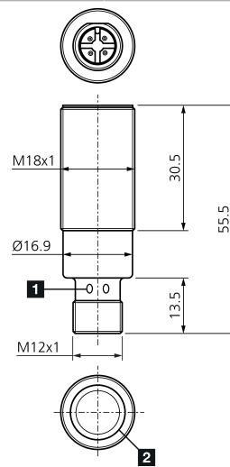
1) LED 2 x 2 / LED 2 x 2 / LED 2 x 2 2) Schallaustritt Ultraschallwandler / Sound outlet ultrasonic transducer / Sortie sonore transducteur à ultrasons mm
